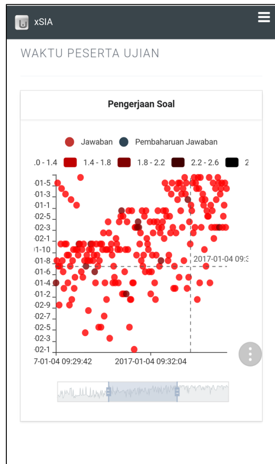
Gambar 10. Pola Jawaban Peserta Ujian
